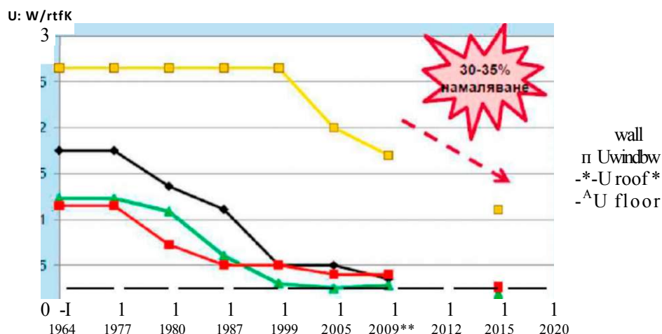
Фиг. У9-2: Предложение за подобряване на енергийните характеристики на сградните ограждащи конструкции и елементи
