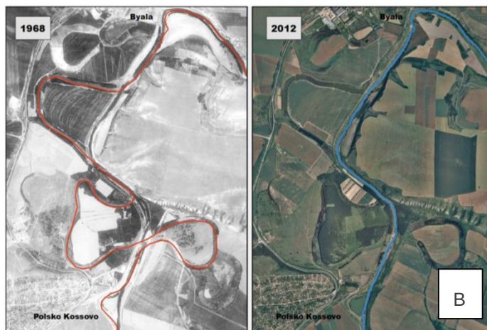
Фигура 10: Участък на заливна равнина (маркиран в ярко синьо) с висок потенциал за намаляване на риска от наводнения, по-специално за подробен параметър „Характеристики на заливната равнина (А.5)“ (А) в сравнение с предишното изправено речно корито с откъснати меандри на р. Янтра (В, взето от INTERREG (INTERREG – DANUBE TRANSNATIONAL PROGRAMME 2020))
