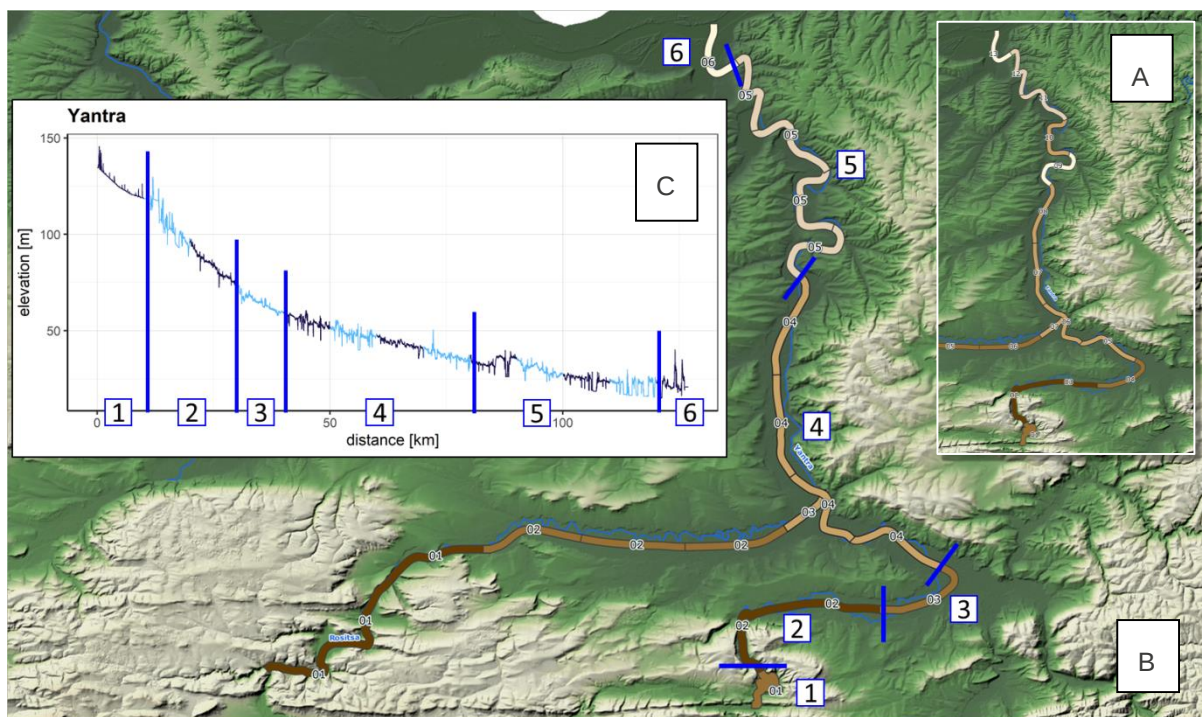
Фигура 5: Категории на наклона в участъците от заливната равнина с дължина 10 km (A), агрегирани типове заливни равнини с хомогенни условия по отношение на наклона (B) и надлъжен профил на заливната равнина, визуализиращ хомогенните участъци (C) от голям участък от р. Янтра (Участъците в синьо и в черно от надлъжния профил, респективно кодовете на картата, показват анализираните 10 km участъци от заливната равнина).
